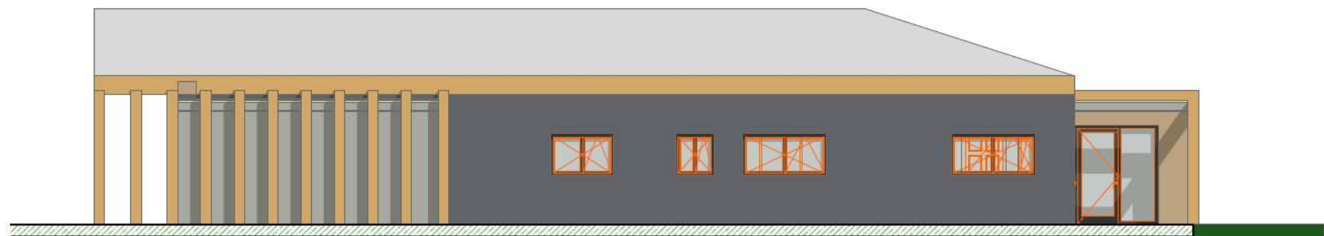
pohled severní
