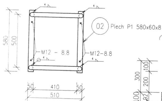
PŮDORYS ZÁKLADU
