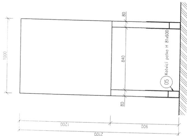
POHLED ČELNÍ
