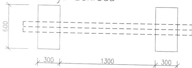
Půdorys základu
