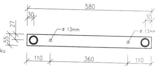
PLECH P1
