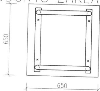
VÝROBNÍ VÝKRES
