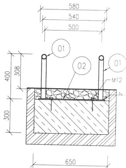
PLECH P1
