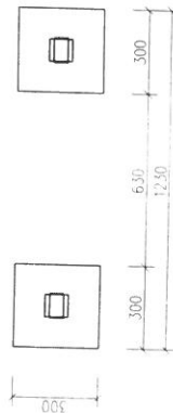
PŮDORYS ZÁKLADU
