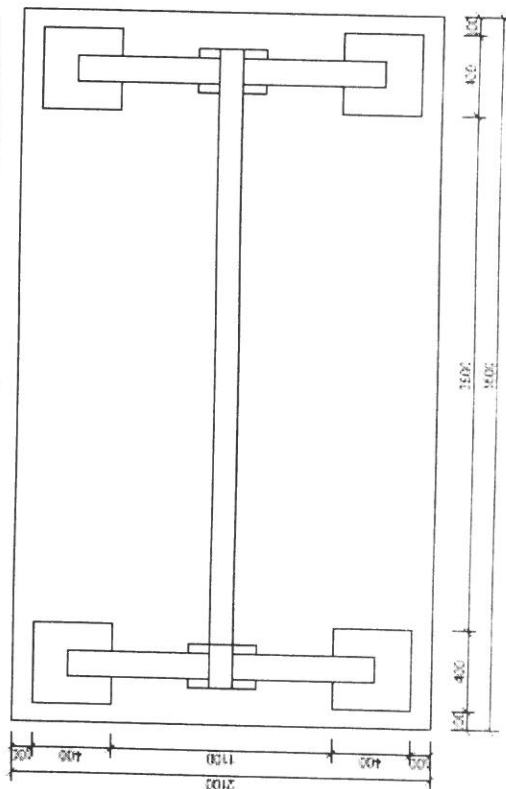
PŮDORYS ZÁKLADU
