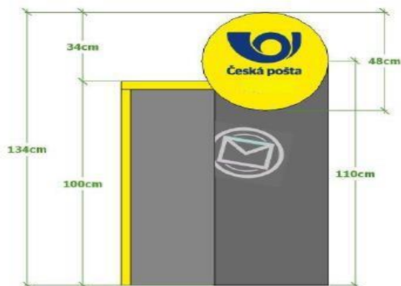
POHLEDY:
